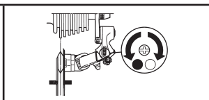
Рис. 18: Регулировка заднего переключателя, установка нижнего предела (вид на переключатель сзади)
