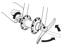
Рис. 9: Эксцентрикый зажим колеса
