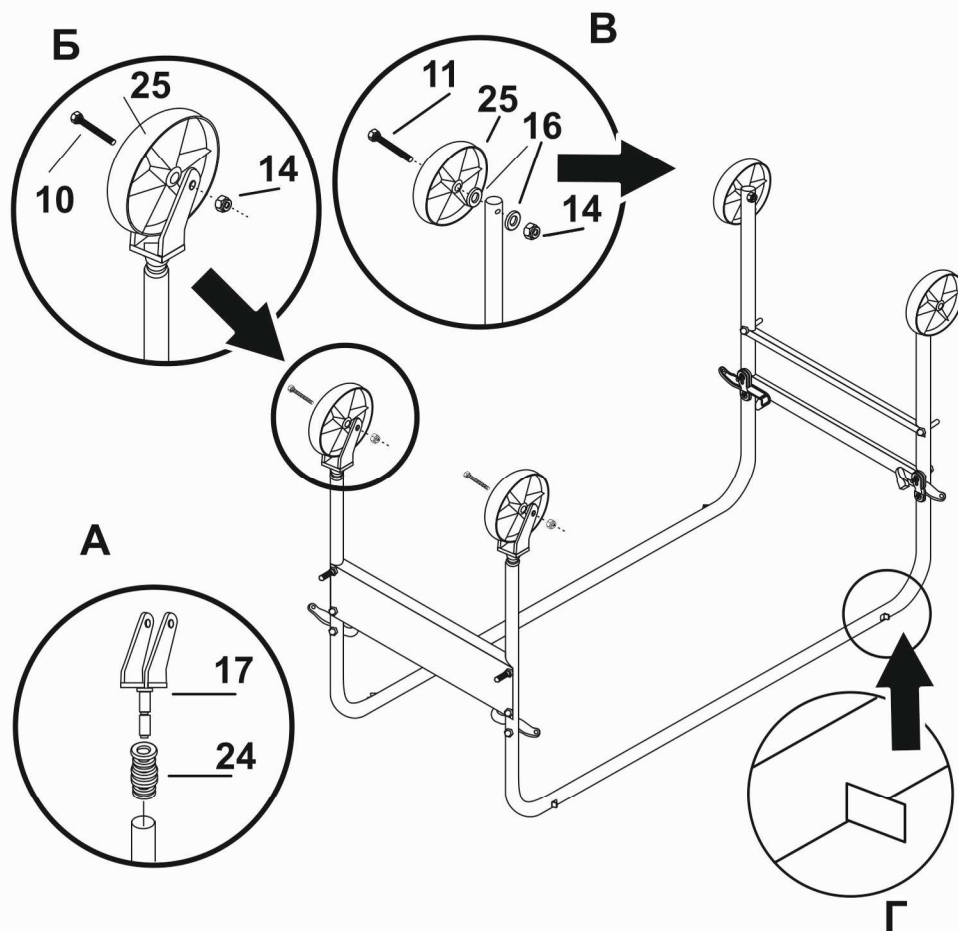
Сборка колес. Рис. 3
