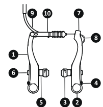
13.2-сур.: V-типті тежегіш және оның реттемелері
