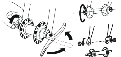
9-сур.: Дөңгелектің эксцентрілі қысқышы
