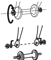
10-сур.: Дөңгелекті сомын арқылы бекіту
