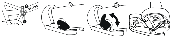
29-сур.: Арзан жиналмалы велосипед қаңқасының құрылысы: 1. Эксцентрик иінітпегі; 2. Құлып қорысқы. 30-сур.: Жиналмалы велосипед қаңқасының құлып жабық күйде, сақтандырғыш бұғатталған. 31-сур.: Жиналмалы велосипед қаңқасының құлып жабық күйде, сақтандырғыш ашылған. 32-сур.: Жиналмалы велосипед қаңқасының құлып ашық күйде, велосипед қаңқасы жиналған.
