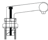
26-сур.: Бұрамалы руль бағанының конструкциясы және руль қалпын реттеуі
