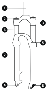
27-сур.: Велосипед амортизациялық ашаның конструкциясы
