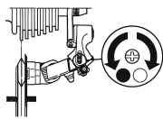
18-сур.: Артқы ауыстырып қосқышты реттеу, төменгі шекті орнату (ауыстырып қосқыштың артқы керілісі)
