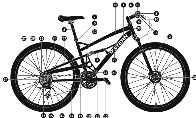
1-сур.: Заманауи тау велосипедінің құрылымы
