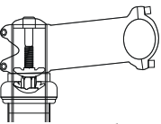
25-сур.: Бұрамалы руль бағанының конструкциясы және шығарым реттеуі
