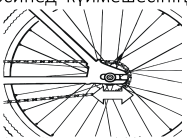
24-сур.: Шынжыр керілісін өзгерту үшін қаңқа дропауттарындағы артқы дөңгелек осін жылжыту керек.
